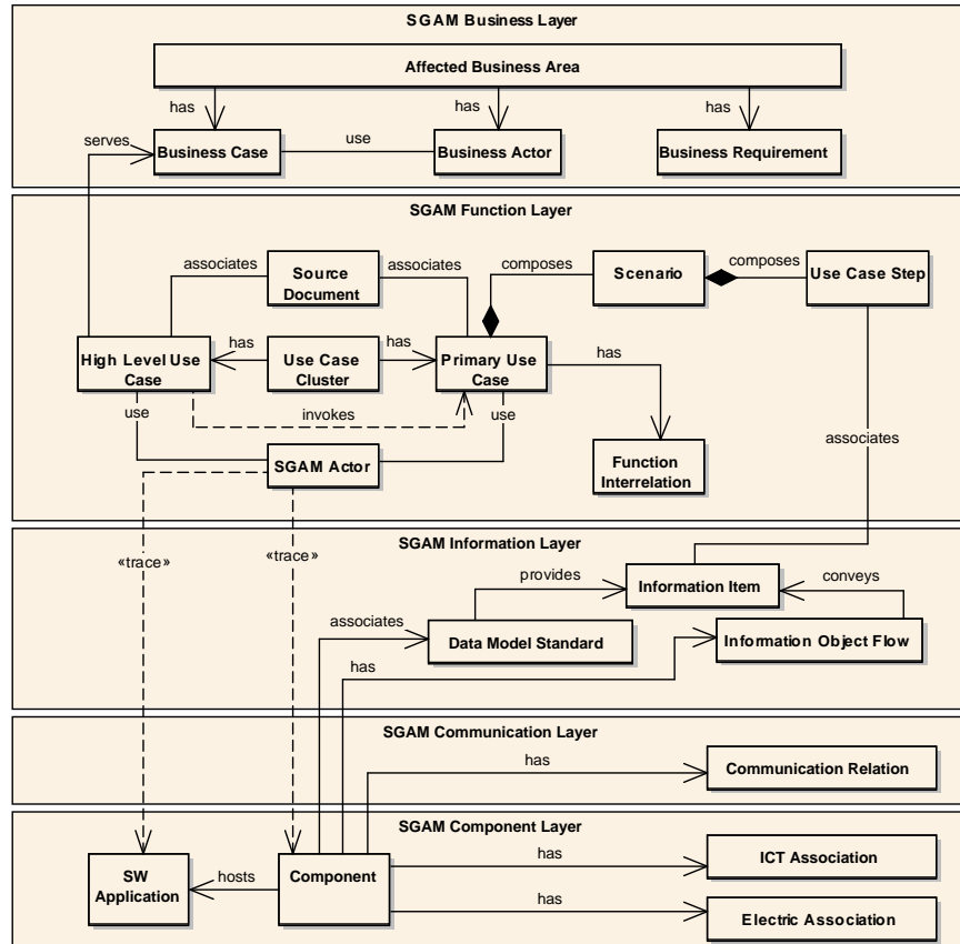
Fig. 3 The INTEGRA Meta-model
